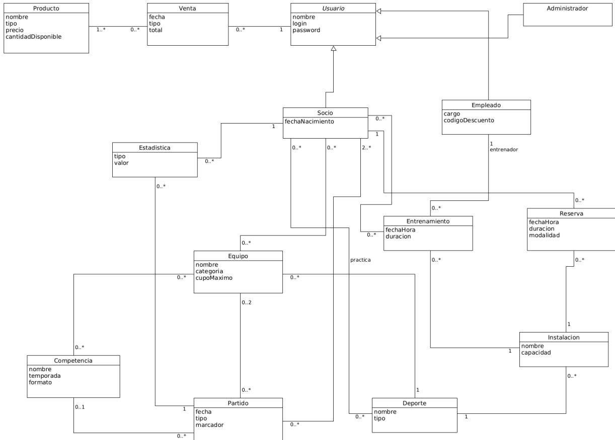
Club Deportivo Séneca - Modelo de dominio
